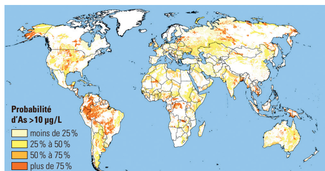
Probabilité d'occurrence d'eaux souterraines présentant des concentrations d'arsenic supérieures au seuil de 10µg/L fixé par l'OMS. (Amini et al. 2008b)
