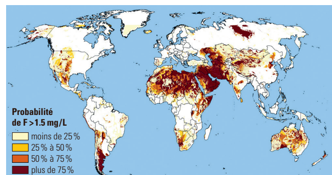
Probabilité d'occurrence d'eaux souterraines présentant des concentrations de fluor supérieures au seuil de 1.5mg/L fixé par l'OMS. (Amini et al. 2008a)
