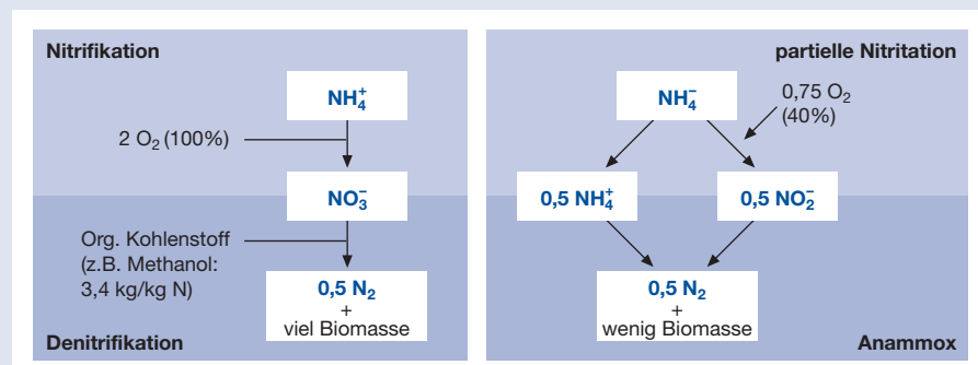
Abb. 3: Vergleich des Anammox-Verfahrens (rechts) mit der konventionellen Stickstoffeliminierung durch das Nitrifikation/Denitrifikations-Verfahren (links).
