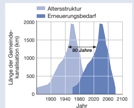
Abb. 2: Altersstruktur der Kanalisation im Kanton Bern [4].
