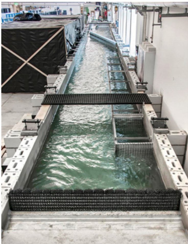
Versuchskanal an der VAW/ETH-Hönggerberg (Foto: VAW)
