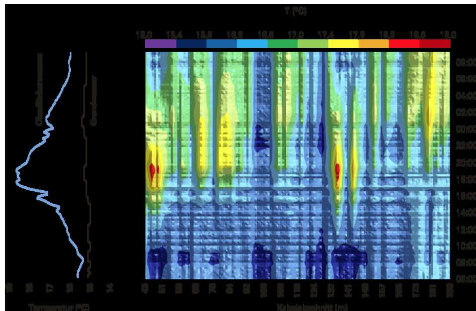
Abb. 3: Temperaturmessung im Chriesbach (ZH) im Sommer 2014 von morgens 6 Uhr bis am nächsten Tag 9 Uhr. Die Kurven links stellen die Temperatur des Oberflächenwassers (hellblau) und des Grundwassers (schwarz) dar. Die Darstellung rechts gibt die Temperaturen wieder, die mit dem im Bachbett verlegten, rund 150 Meter langen Glasfaserkabel gemessen wurden. Gut zu sehen ist, dass es Bereiche gibt, wo kaum warmes Flusswasser am Kabel vorbei ins Grundwasser strömt (z.B. Abschnitt von 95 bis 105 Meter), und andere, wo sich der oberflächliche Tagesgang der Temperatur deutlich im Bachgrund fortsetzt (z.B. bei 47 Meter und 137 Meter).
