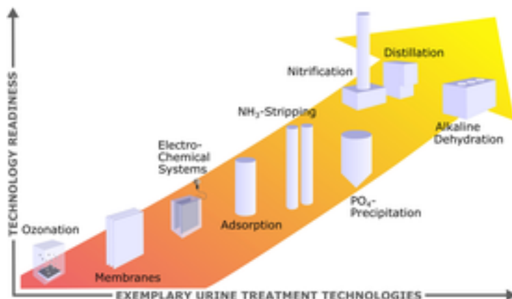
Verschiedene Wege zur Urinbehandlung und deren gegenwärtige Praxisnähe. (Grafik: Eawag)
