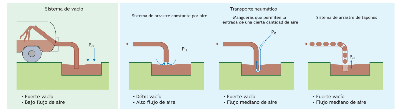
Figura 4.9 Cuatro tipos de técnicas para aspirar los lodos (adaptado de Böesch y Schertenleib, 1985)
