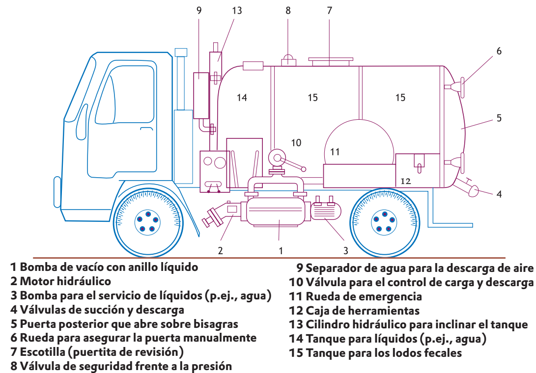
Figura 4.10 Esquema del camión aspirador BREVAC (adaptado de Böesch y Schertenleib, 1985)
