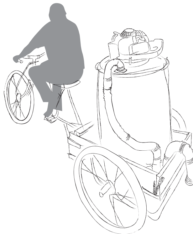
Figura 4.14 Dibujo esquemático de una tecnología para el transporte de lodos fecales impulsada por la fuerza humana (figura: Research Triangle Institute).
