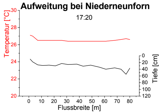
Abbildung 10: Querprofile der Wassertemperaturen in der Thur gemessen am 9. Juli 2003 zwischen 12:45 und 17:20 Uhr. (Distanzen vom rechten Flussufer gemessen, Temperaturen in roter, Wassertiefen in schwarzer Farbe).
