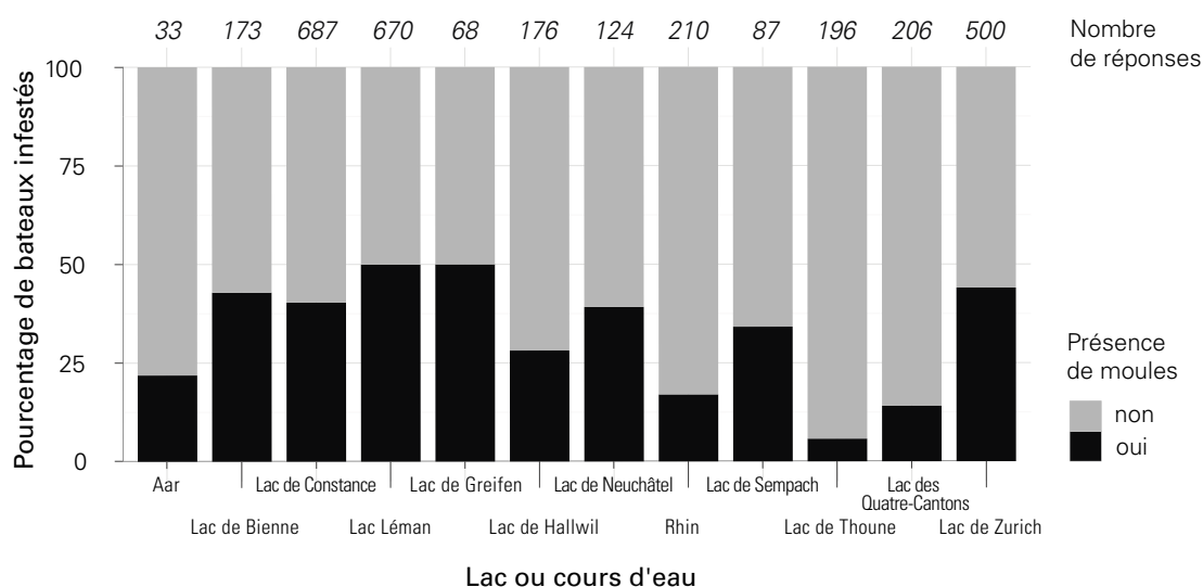
Fig. 3. Pourcentage de bateaux colonisés par les moules (en noir) et nombre de réponses de propriétaires dans chaque lac ou cours d'eau.
