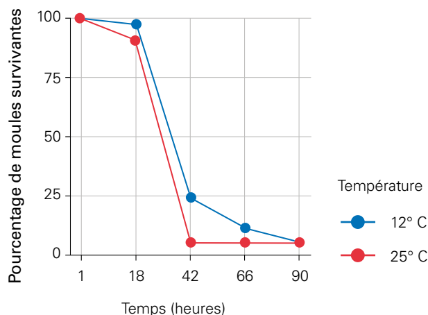
Fig. 7. Pourcentage moyen de moules survivantes au bout de 18, 42, 66 et 90 heures à 12 °C (en bleu) et à 25 °C (en rouge).
