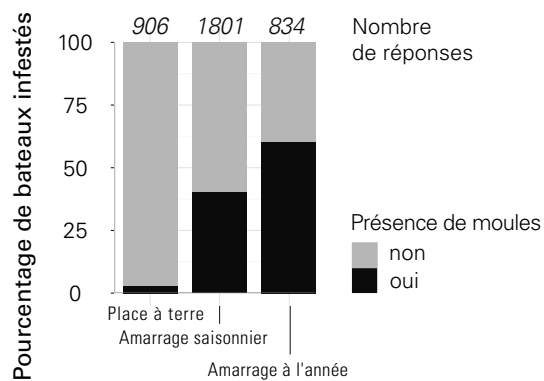
Fig. 4. Pourcentage de bateaux infestés par les moules (en noir) selon le lieu de stationnement (à terre, dans l'eau de façon saisonnière, dans l'eau à l'année).
