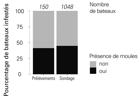
Fig. 5. Les résultats des prélèvements directs sur la coque des bateaux (dans 5 lacs) confirment ceux du sondage corrélatif.
