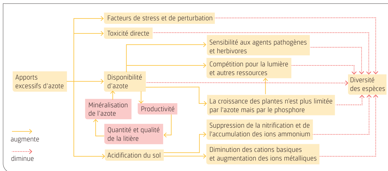
Fig. 3: Incidences des apports excessifs d'azote sur la diversité des espèces. Adapté de Dise et al. (2011) 70 in The European Nitrogen Assessment; 24 reproduit avec l'autorisation de Cambridge University Press via PLSclear.
