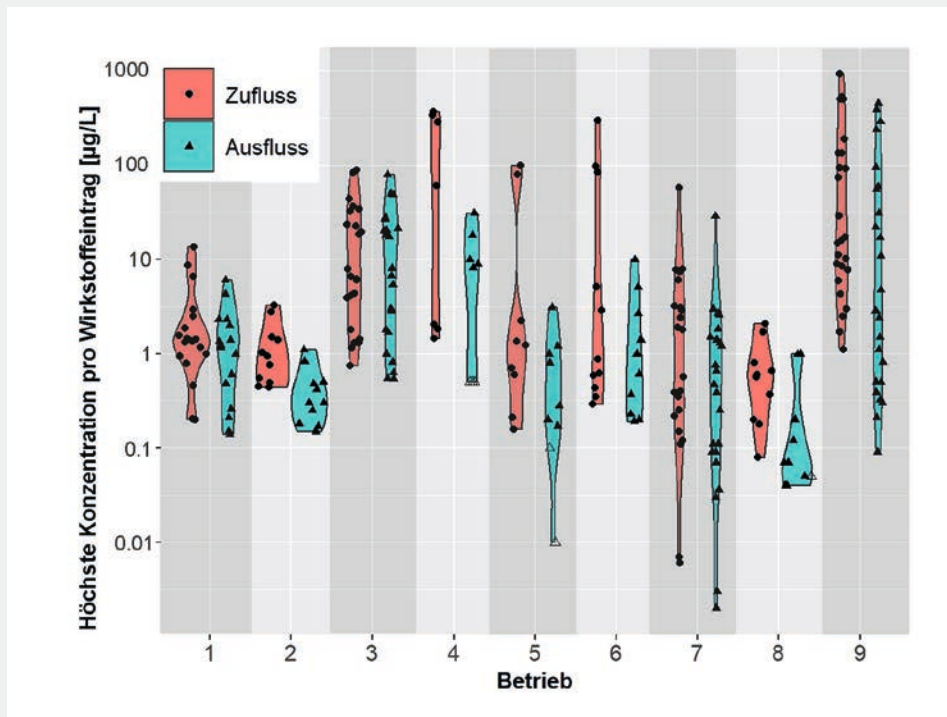
Fig. 4 Höchste gemessene Konzentrationen im Zu- und Ablauf jedes pulsartigen Werkstoffeintrags, verursacht durch die Einleitung von Betriebsabwasser. Nicht gefüllte Symbole zeigen die Bestimmungsgrenze für Substanzen mit Pulseintrag, die im Auslauf nicht mehr zuverlässig quantifiziert werden konnten.
