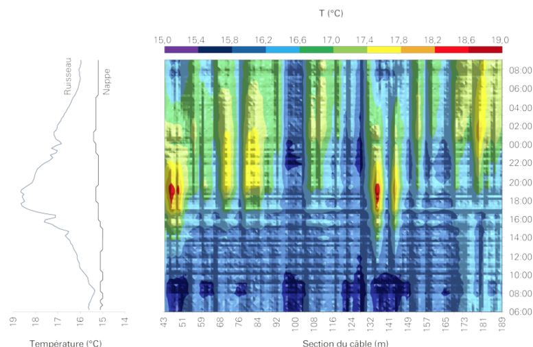
Fig. 3 : Mesures de température dans le Chriesbach (ZH) effectuées pendant l'été 2014 d'un jour à 6 heures du matin au lendemain 9 heures. Les lignes de gauche indiquent l'évolution de la température dans le ruisseau (en bleu clair) et dans la nappe (en noir). L'image de droite correspond aux températures mesurées le long du câble de fibre optique de 150 m de longueur enfoui dans le lit du cours d'eau. On distingue nettement des zones dans lesquelles le flux d'eau réchauffée s'infiltrant dans le sous-sol en passant à côté du câble est quasiment inexistant (entre 95 et 105 cm, notamment) et d'autres dans lesquelles la température dans le lit évolue parallèlement à celle mesurée dans le ruisseau (à 47 m et à 137 m par exemple).
